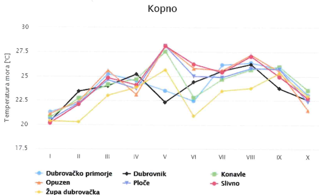
Graf 7. Prosječna temperatura mora na morskim plažama u Dubrovačko-neretvanskoj županiji po ispitivanju na kopnu u 2024. godini
