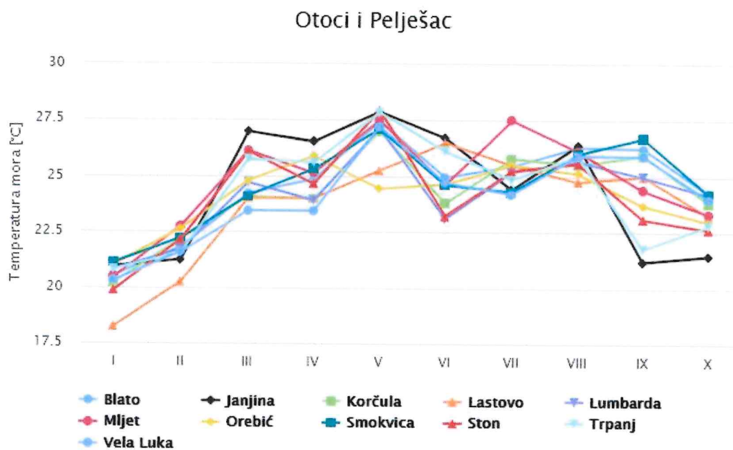
Graf 9. Prosječna temperatura mora na morskim plažama u Dubrovačko-neretvanskoj županiji po ispitivanju na otocima i poluotoku Pelješcu u 2024. godini
