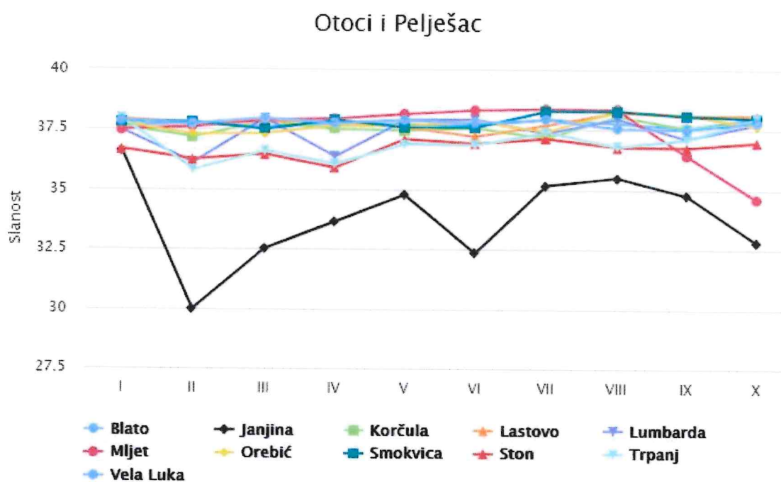
Graf 10. Prosječna izmjerena slanost mora na morskim plažama u Dubrovačko-neretvanskoj županiji po ispitivanju na otocima i poluotoku Pelješcu u 2024. godini
